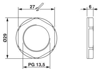
尺寸图
