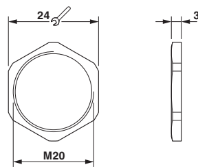
尺寸图
