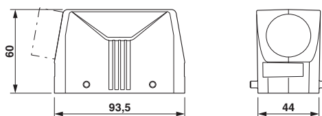
尺寸图
