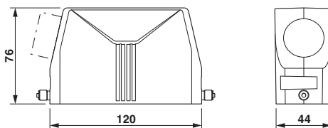
尺寸图
