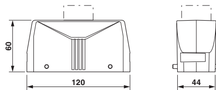
尺寸图
