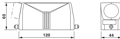
尺寸图
