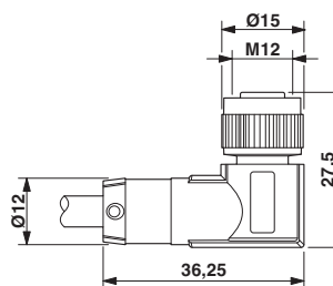
尺寸图
