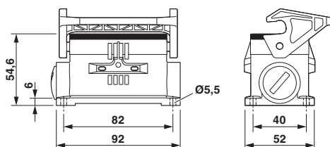
尺寸图
