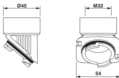
尺寸图
