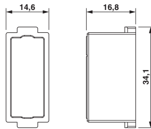
尺寸图
