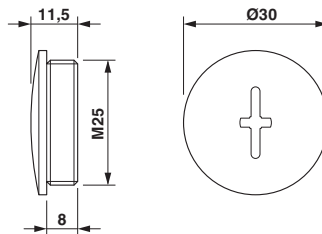
尺寸图
