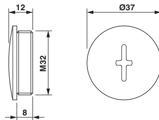
尺寸图
