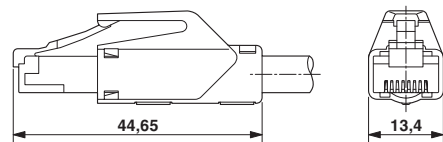
尺寸图
