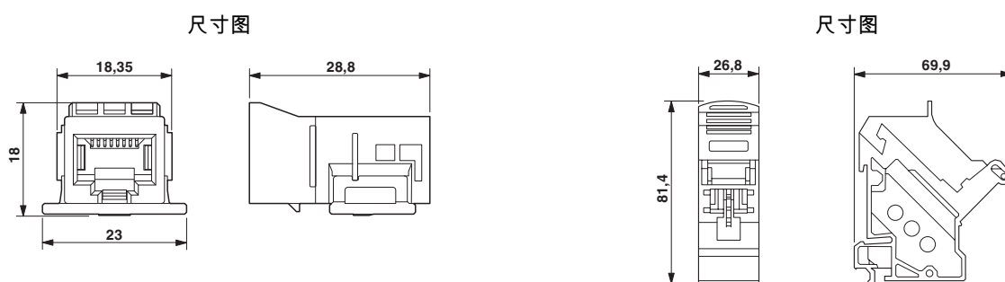
RJ45插座, Freenet连接技术
