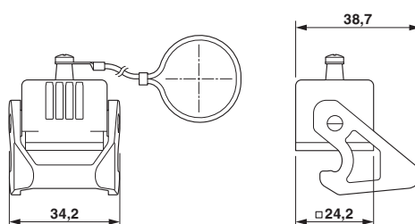
尺寸图
