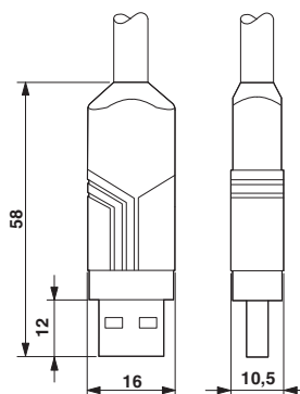
尺寸图
