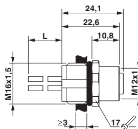
尺寸图
