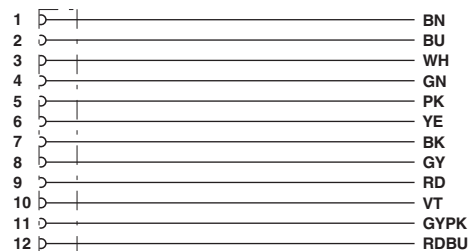
M12孔式触点分配
