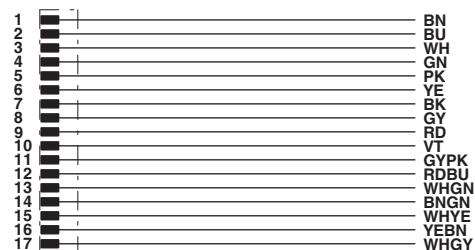
M12针式触点分配
