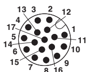
M12针式连接器的引脚分配, 17芯, 插头侧视图
