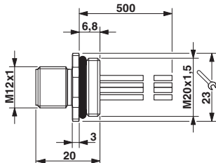
尺寸图
