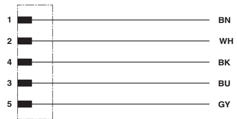
电路图
