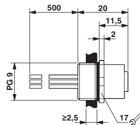
尺寸图
