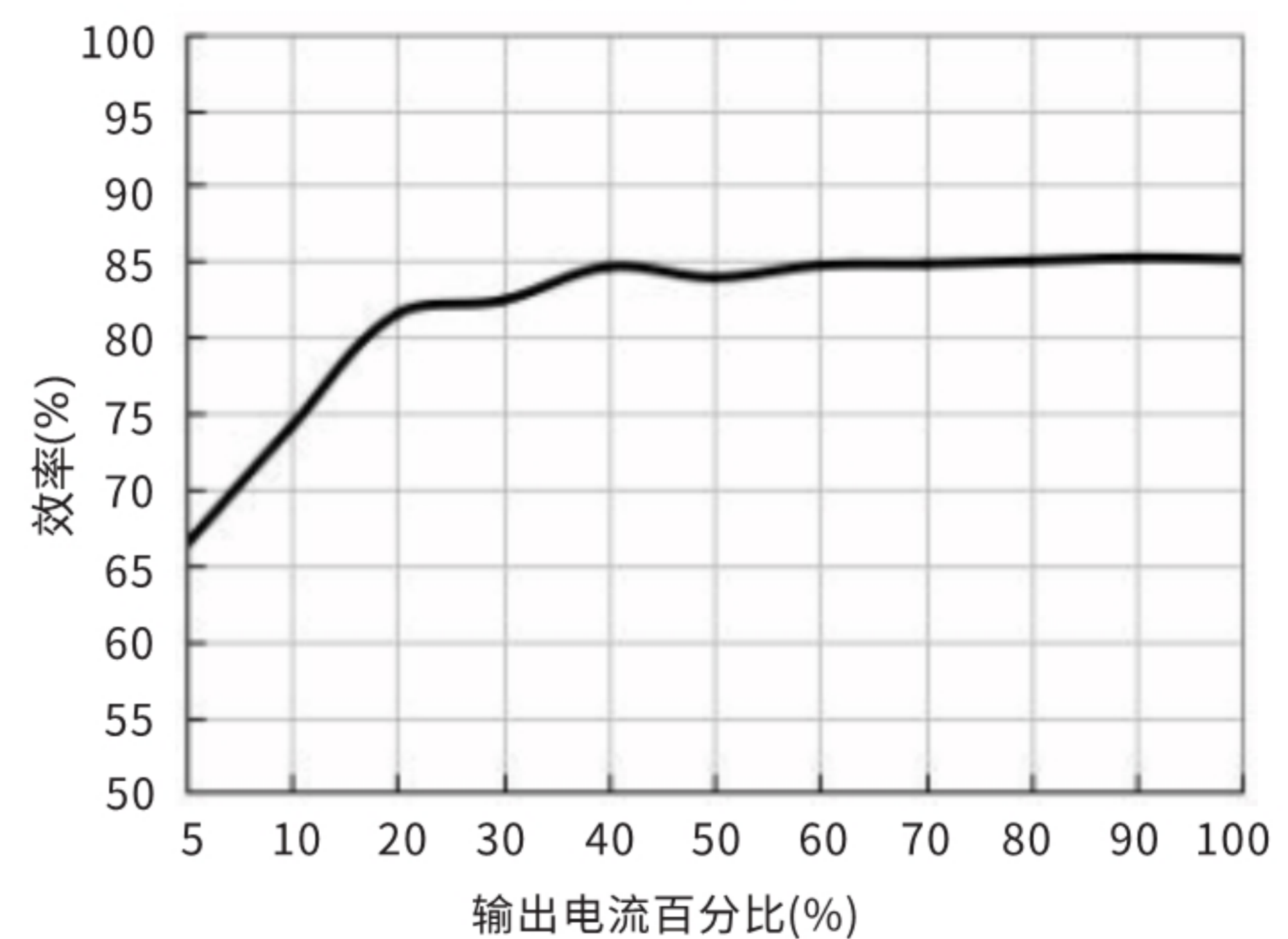
效率Vs输出负载(Vin=24V) URB2405YMD-6WR3
