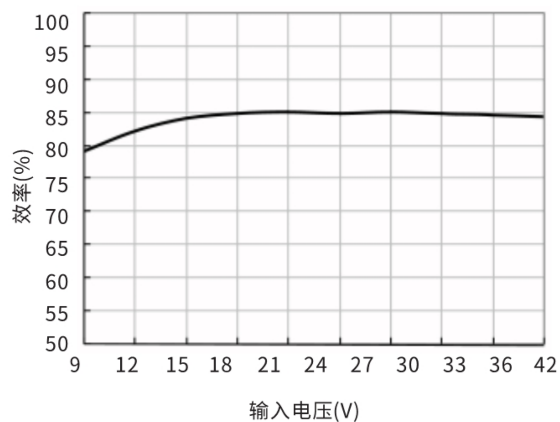
效率Vs输入电压(满载) URB2405YMD-6WR3
